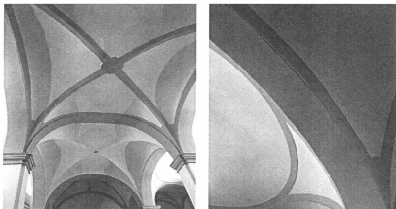
Fisuras en las bóvedas de la nave central
